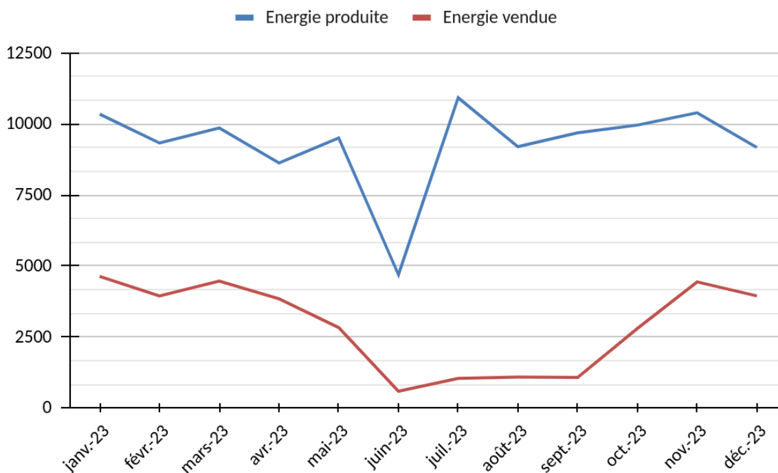
Figure 12 : Énergies thermiques produite et vendue
