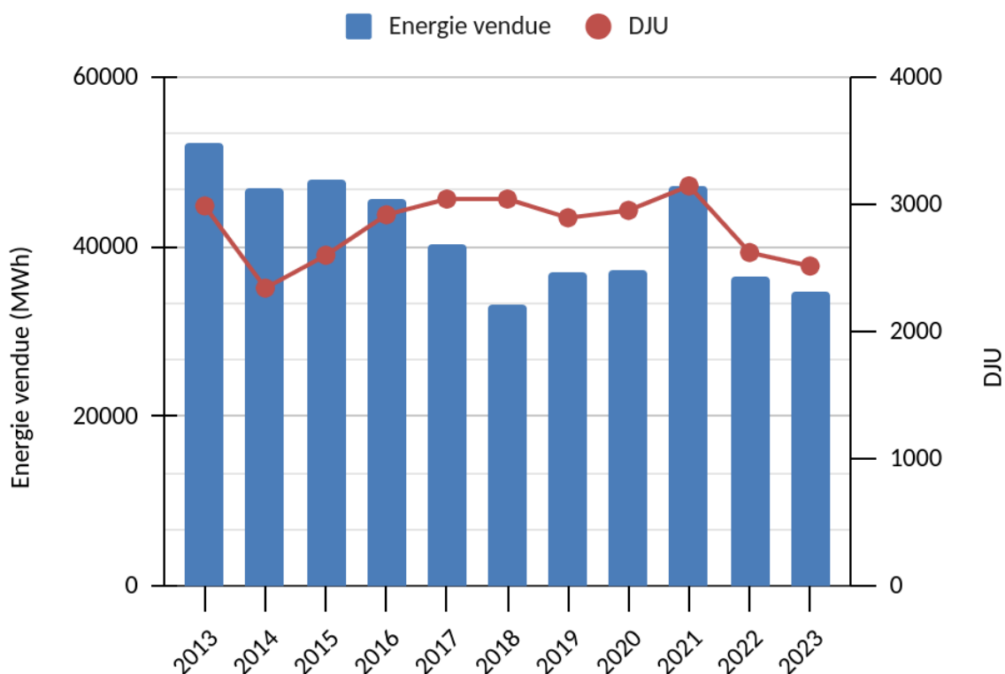
Figure 13 : Énergie vendue et DJU depuis 2009
